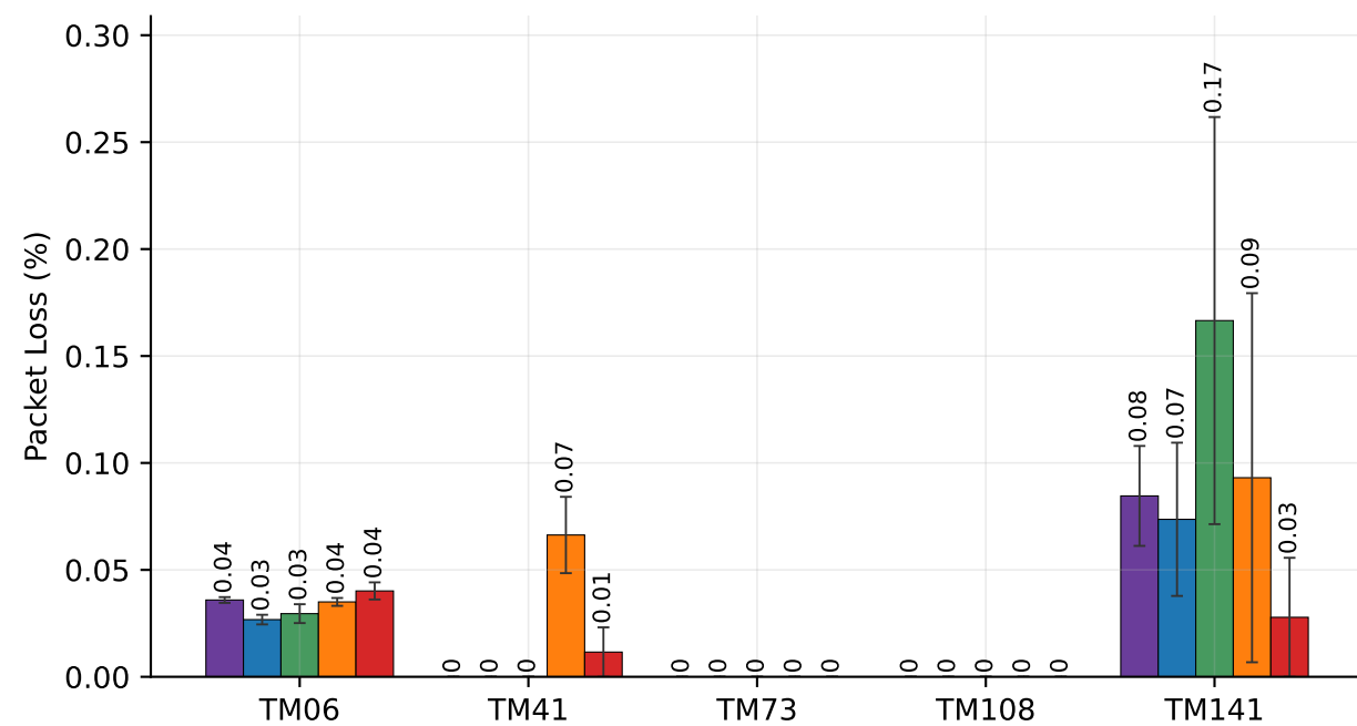
(d) Average Packet Loss ↓
